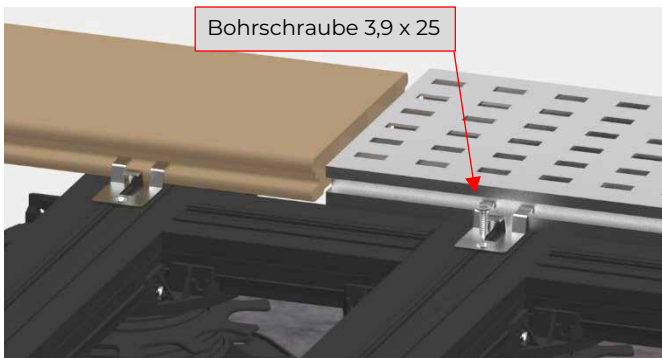
Bild 24. Danach werden die Distanz-Clips auf die WPC-Diele und das Drainageprofil geschoben und mit den Bohrschrauben 3,9 x 25 mm auf der Aluminiumunterkonstruktion geschraubt.
